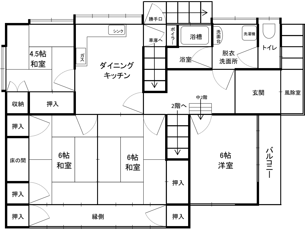
1階 (建物2階)
