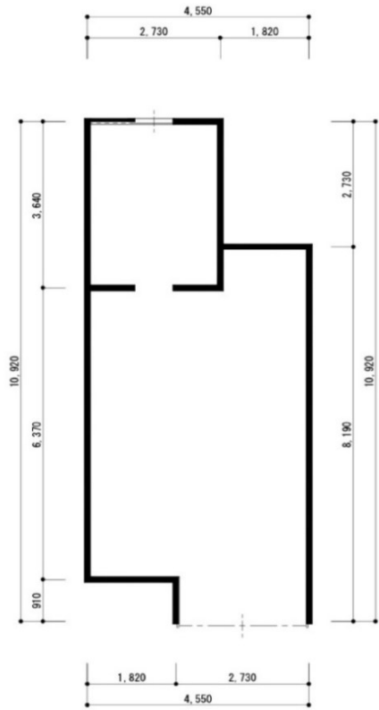
地階平面図 1:100
