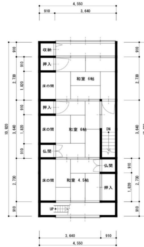
2階平面図 1:100
