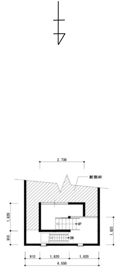
3・4階平面図 1:100
