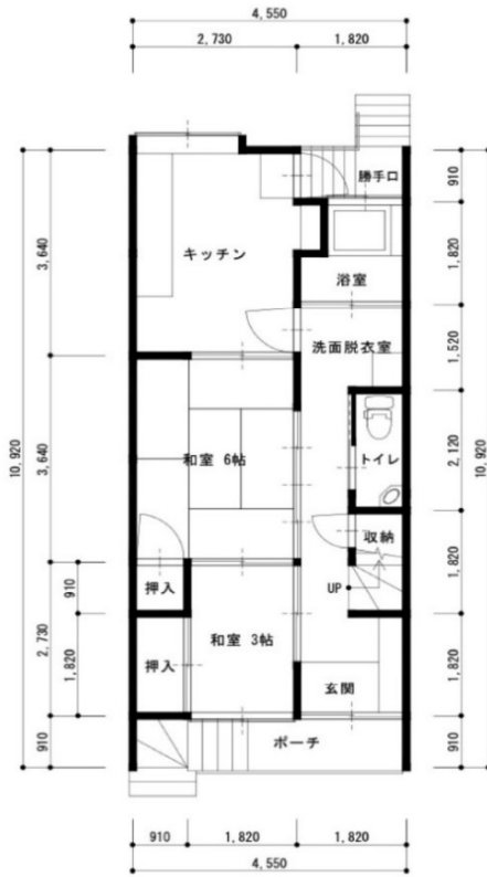
1階平面図 1:100
