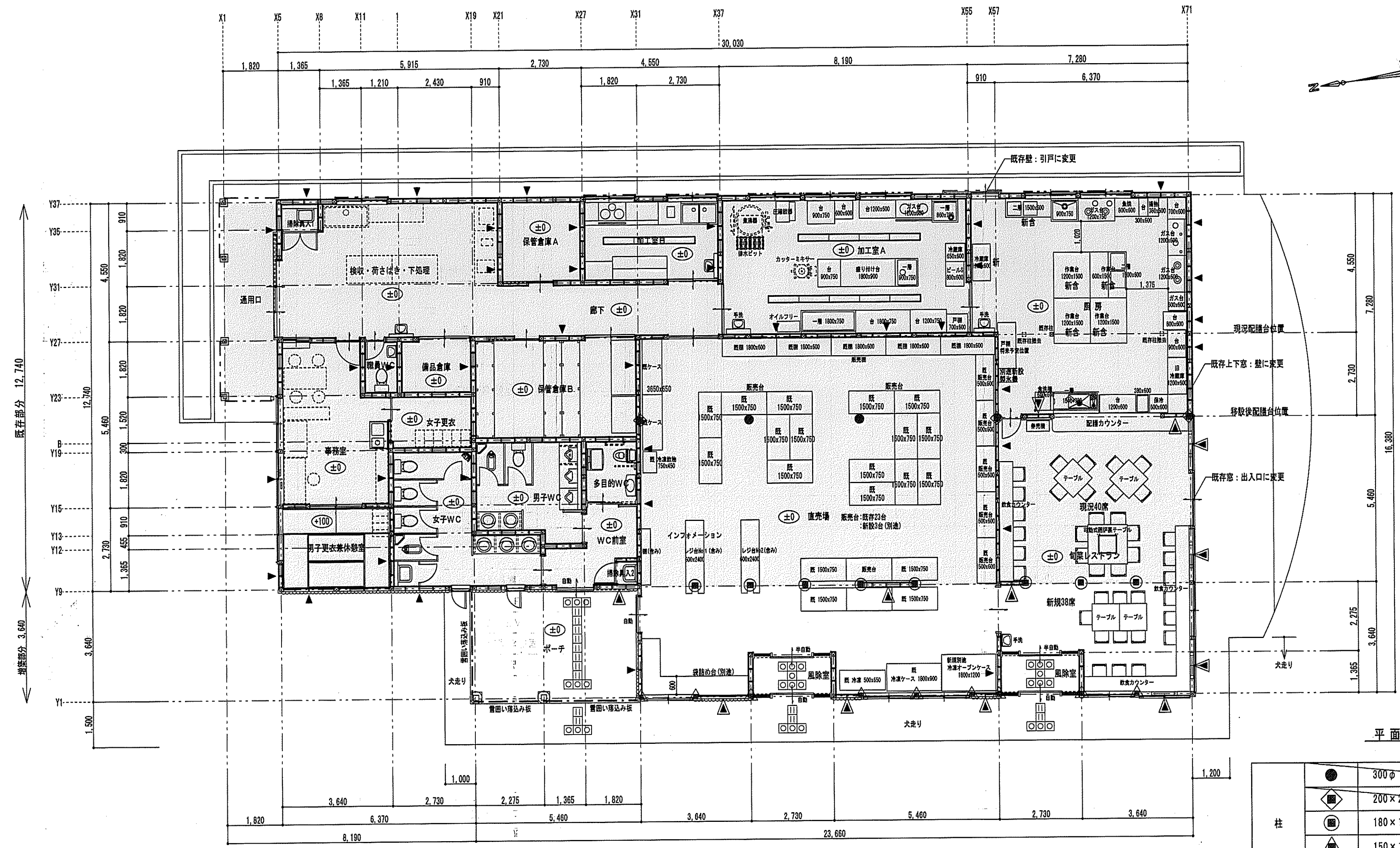
平面図 1:100
