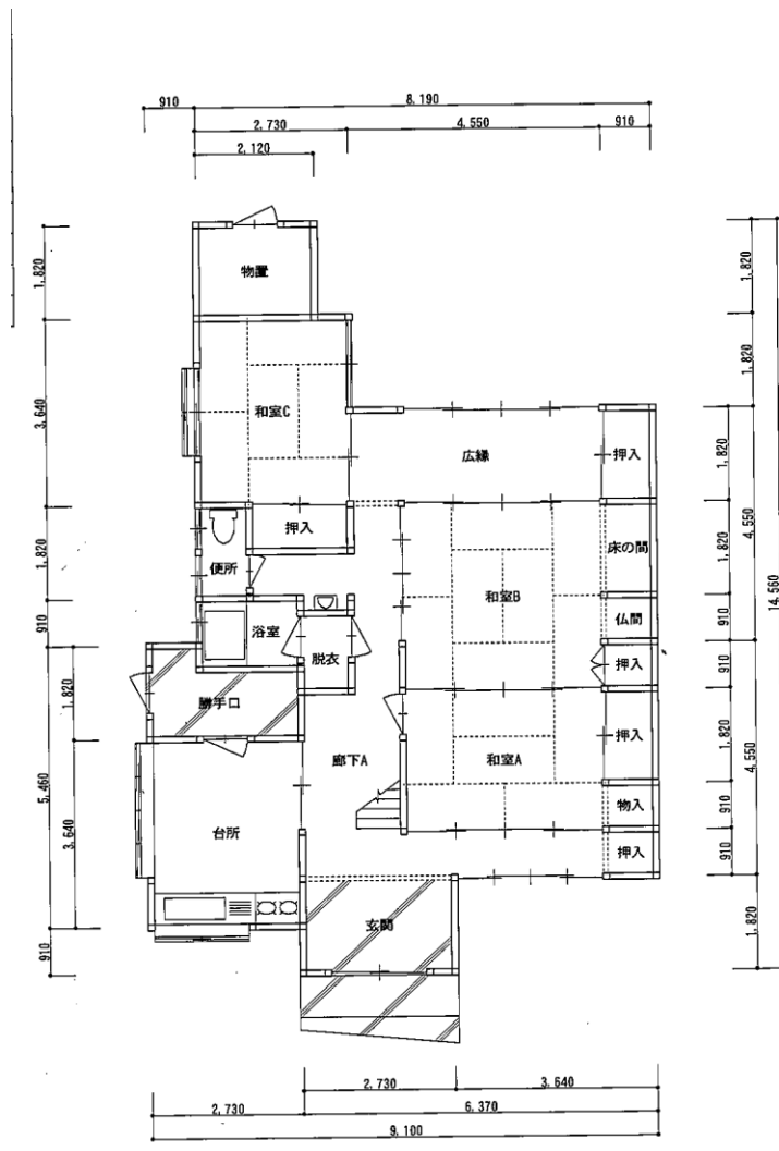
1階 平面図 S=1/100
