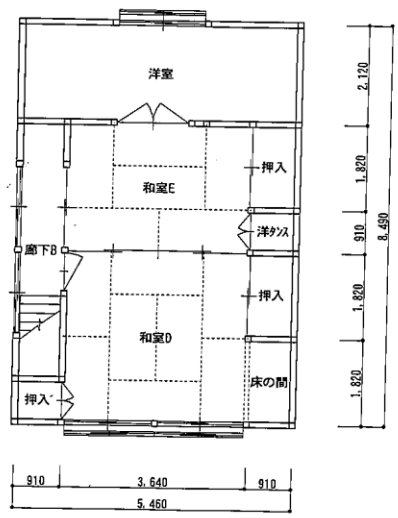
2階 平面図 S=1/100
