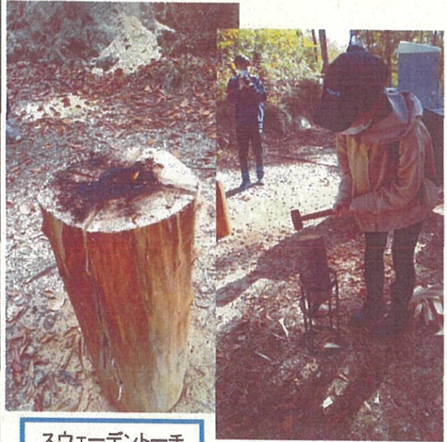
手動薪割り機
