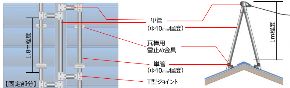
瓦棒用雪止め金具
