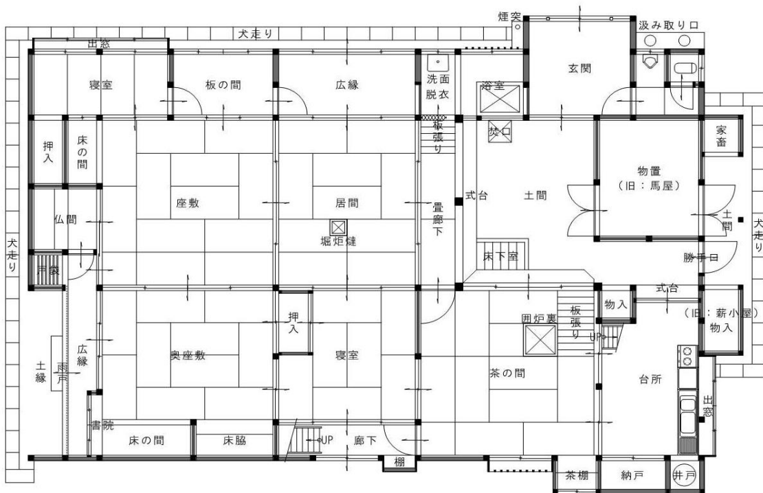
主屋 1階平面図 S=1/100
