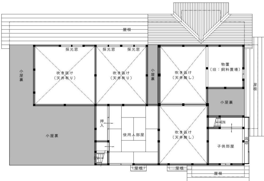
主屋 2階平面図 S=1/100
