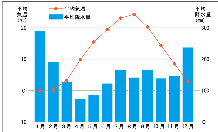
図 2-4 雨温図 (気象庁) 観測地点：関山 統計期間：1987～2016年
